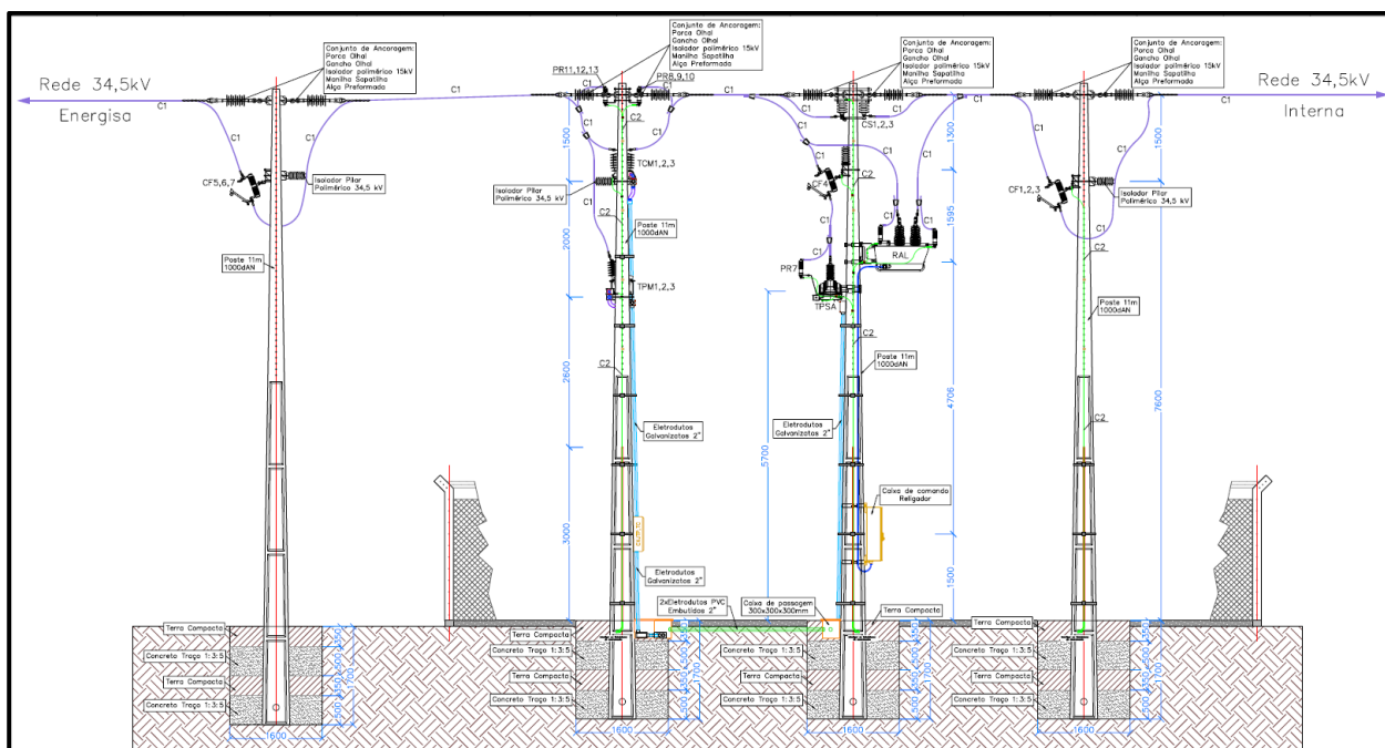
Figura 17: Layout da subestação de energia – Corte Esquemático (extraído do JUR1-02-DE-FE-SE-E20-0002 – REV.00).
